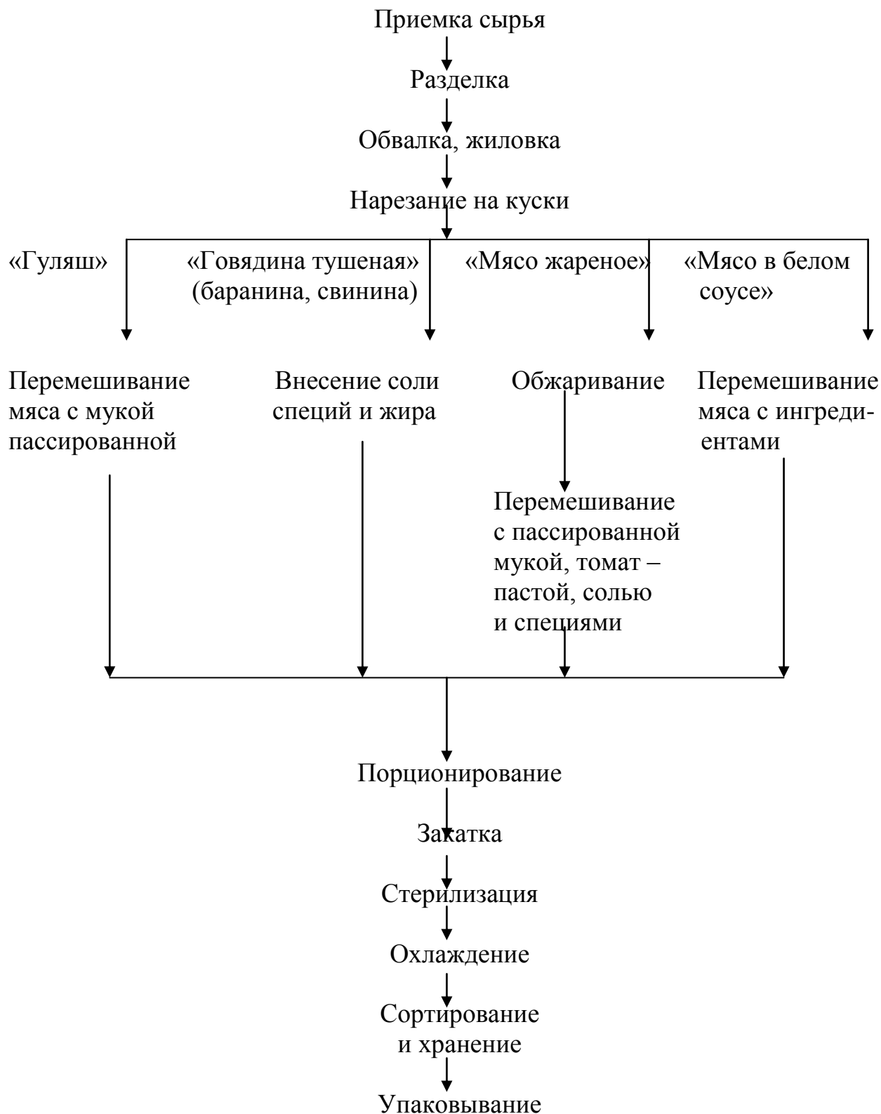
Рис.1.1. Технологический процесс производства натурально-кусковых консервов Приемка мясного сырья
