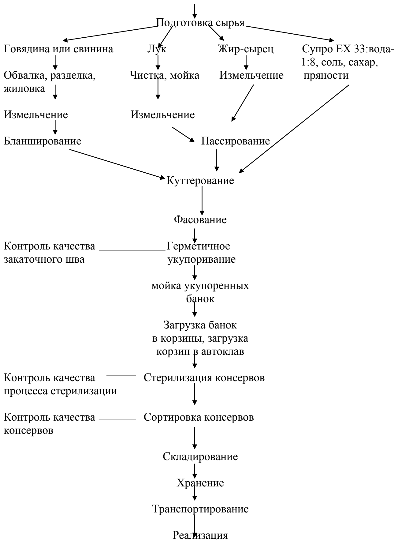
Рис. 1.6. Технологическая схема производства мясных консервов «Паштет для завтрака с мясом» Входной контроль
