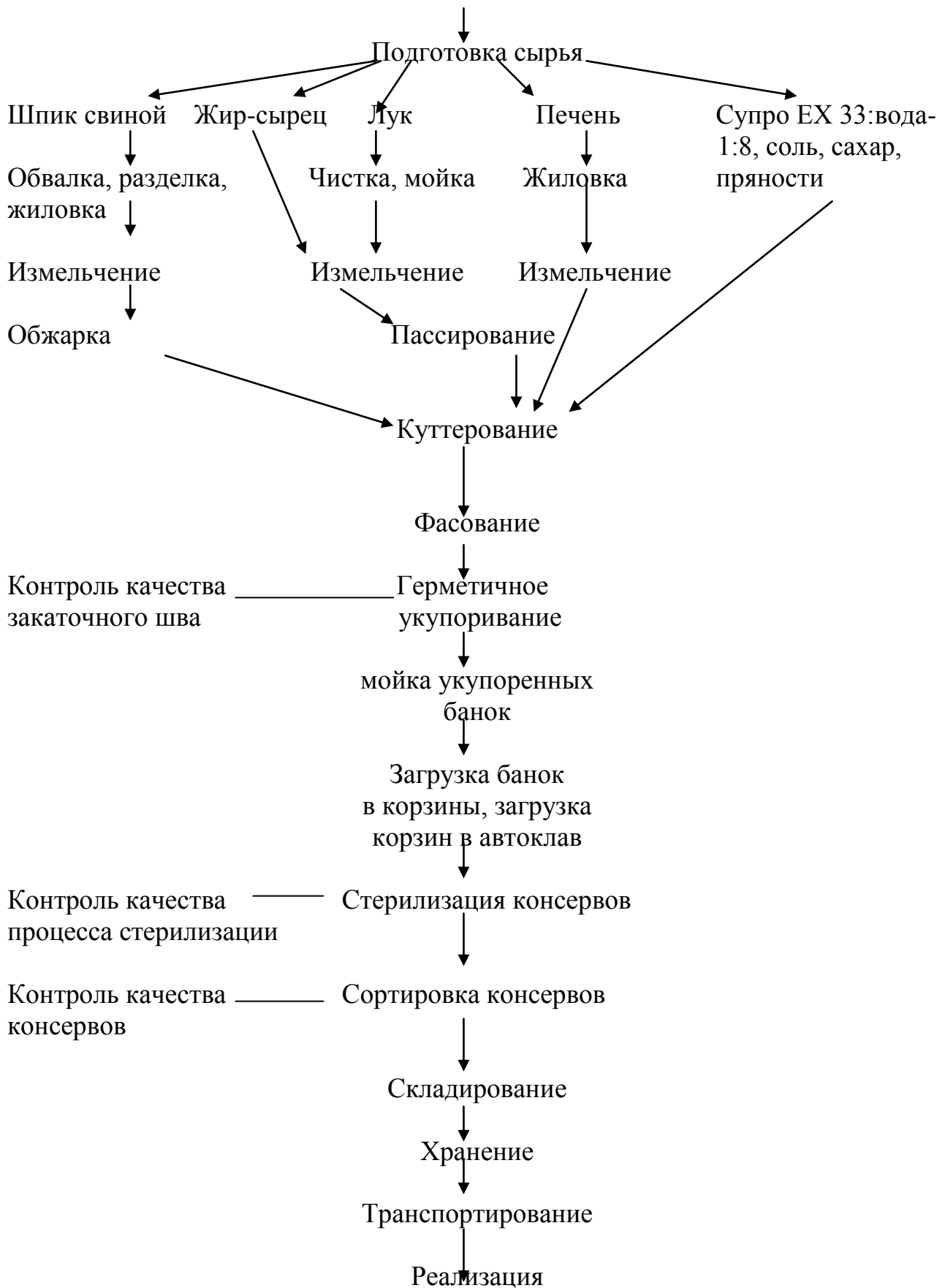
Рис. 1.7. Технологическая схема производства мясных консервов «Крем любительский» Входной контроль
