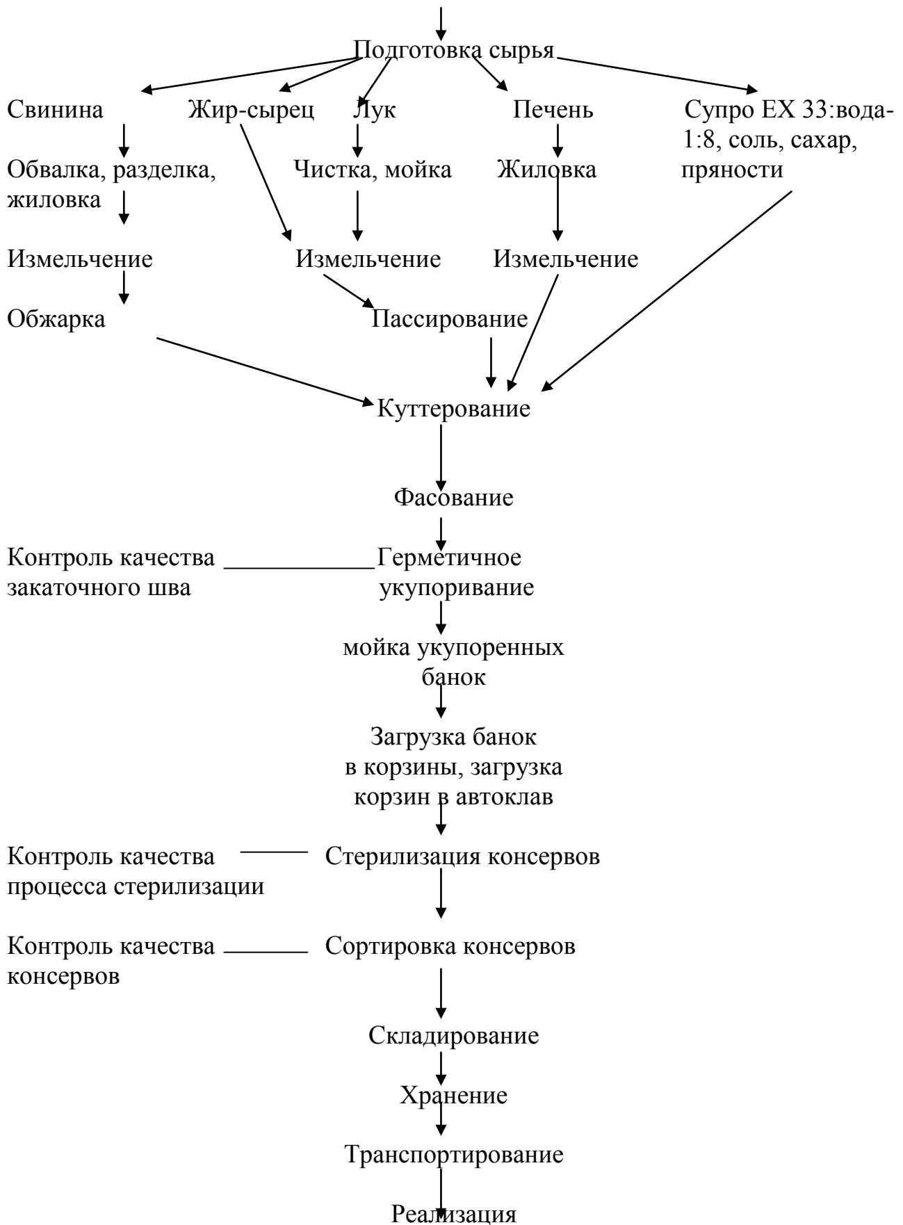
Рис. 1.8. Технологическая схема производства мясных консервов «Паштет для завтрака с печенью» Разделку полутуш (туш) производят как по комбинированной, так и по
